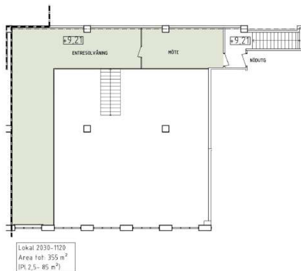
ENTRESOLPLAN
